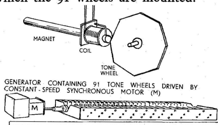
FIG. 95.—Hammond Organ.
